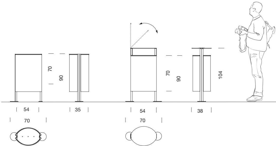
Rambla litterbin 82 litres
